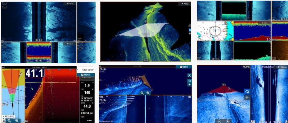
<이미지 소나 구현 화면 (측방, 전방, 하방, 3D 이미지 소나)>
